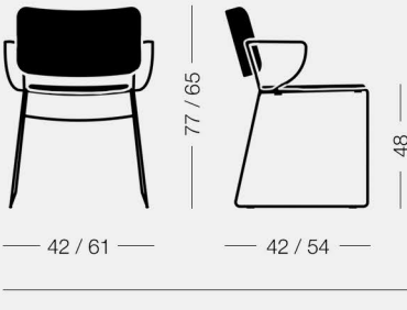
Button Down 7C23 8,1 kg 0,38 m³ 2 pz Poltroncina, sedile e schienale imbottiti Armchair, upholstered seat and backrest
