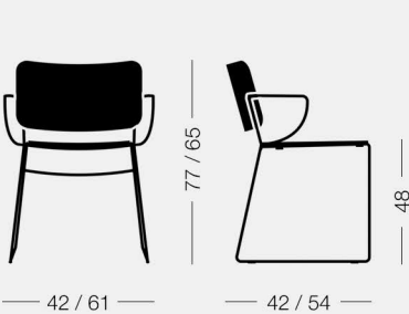
Button Down 7C22 8,1 kg 0,38 m³ 2 pz Poltroncina, sedile e schienale in legno Armchair, wood seat and backrest
