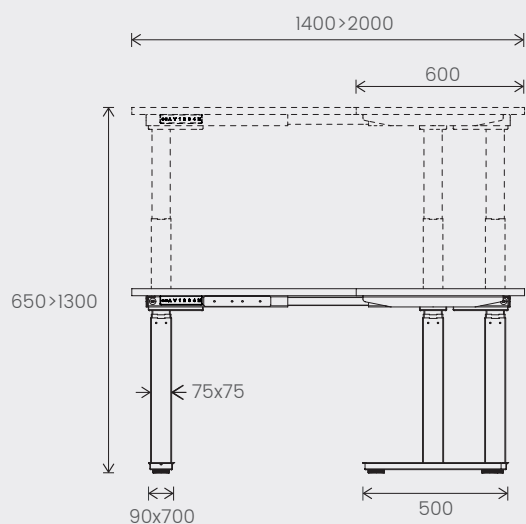
Bureaux structure partagée - Desks with shared structural fram - Bureaus met gedeeld onderstel
